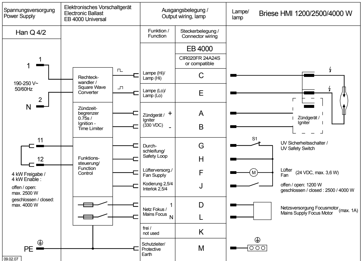
Abb./ Fig. 1: Anschlußbelegung / Connector Wiring
